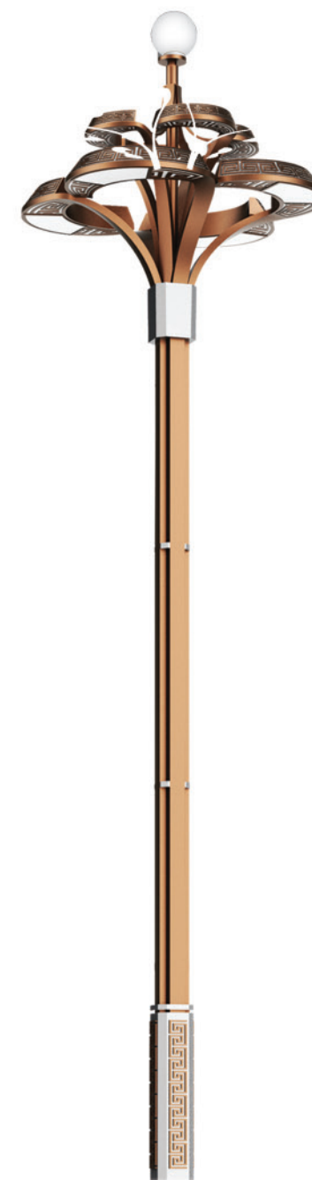
SO-ZH-017 高度 :10-14 米 功率 : 4X120W+9W LED
